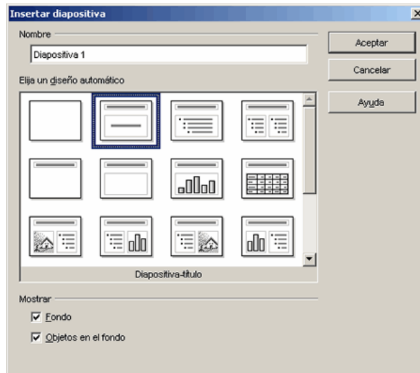
Figura 4: Interfaz diapositiva
